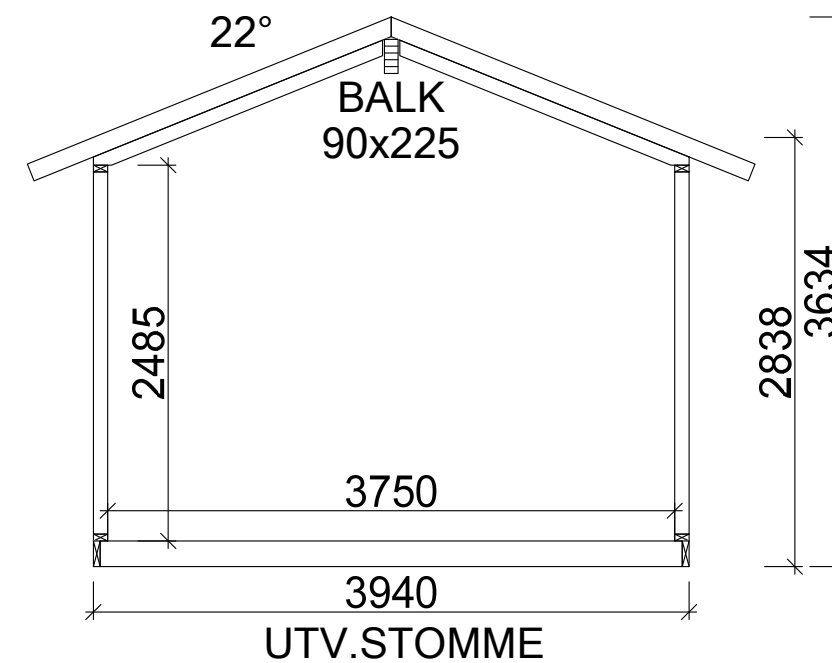
Sektion A-A
