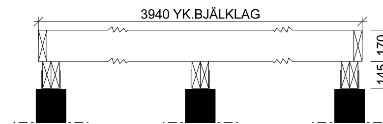
Sektion B-B Skala 1:25
